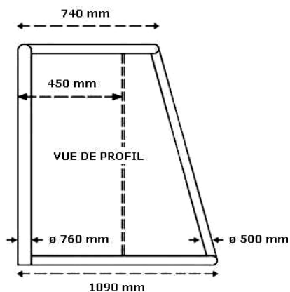
Détail balustrade
